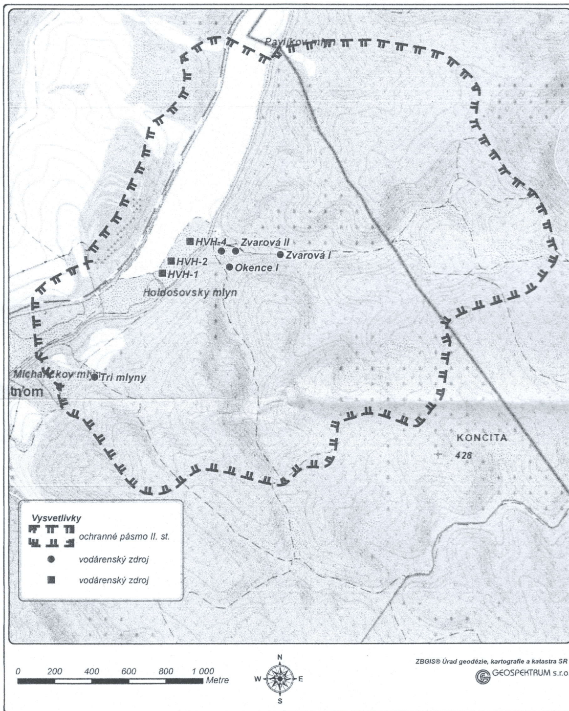
Obr. č. 30 Ochranné pásmo II. stupňa spoločné, na podklade topografickej mapy
